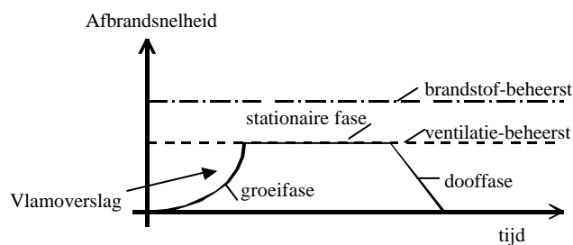
Fig. 4.3: Afbrandsnelheid als functie van de tijd
