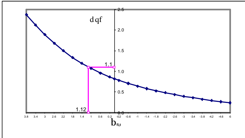
Fig. 5.3: De veiligheidsfactor \delta_{qf} als functie van \beta_{fi,t}
