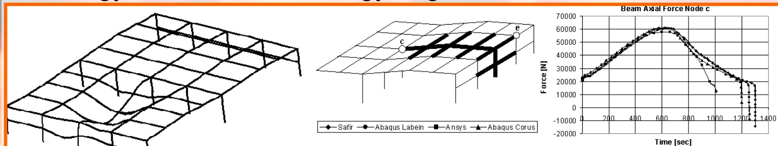
Deformált alak megerősítés nélkül Axiális terhelés
